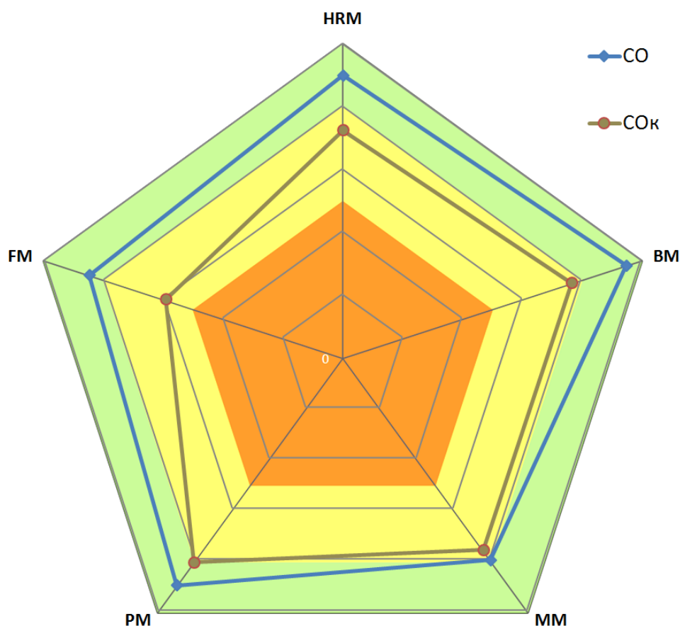
Рис.1. Лепестковая диаграмма: Самооценка (CO), Самооценка скорректированная (COк)
