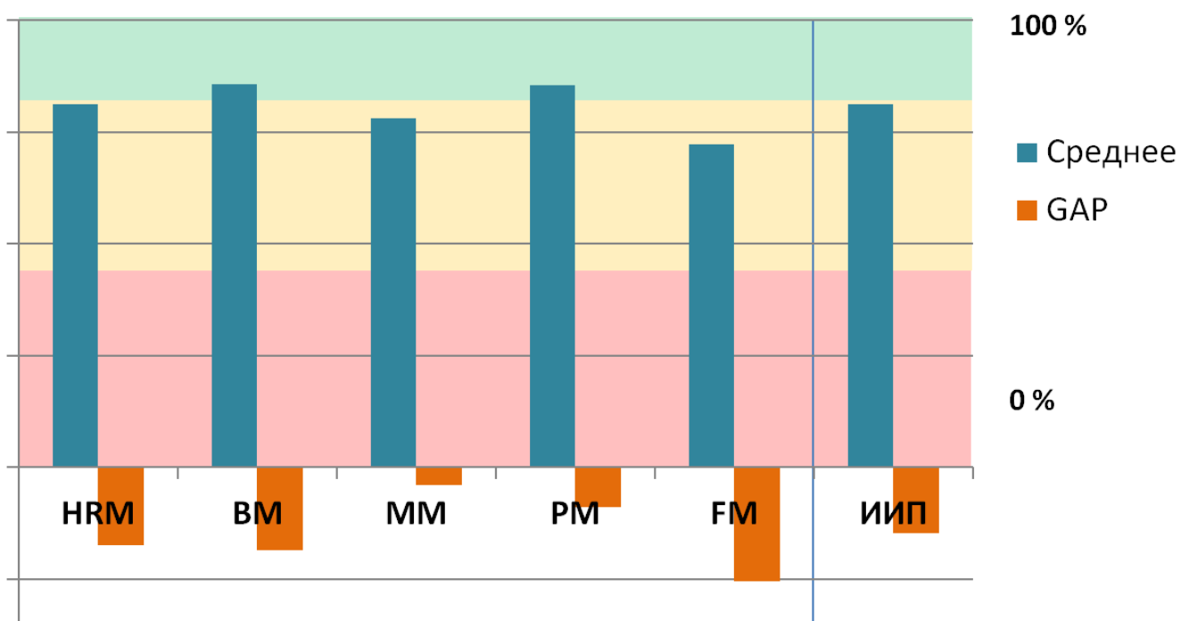
Рис.3. Гистограмма: Среднее = (COк + CO) / 2 , GAP = COк - CO , ИИП
