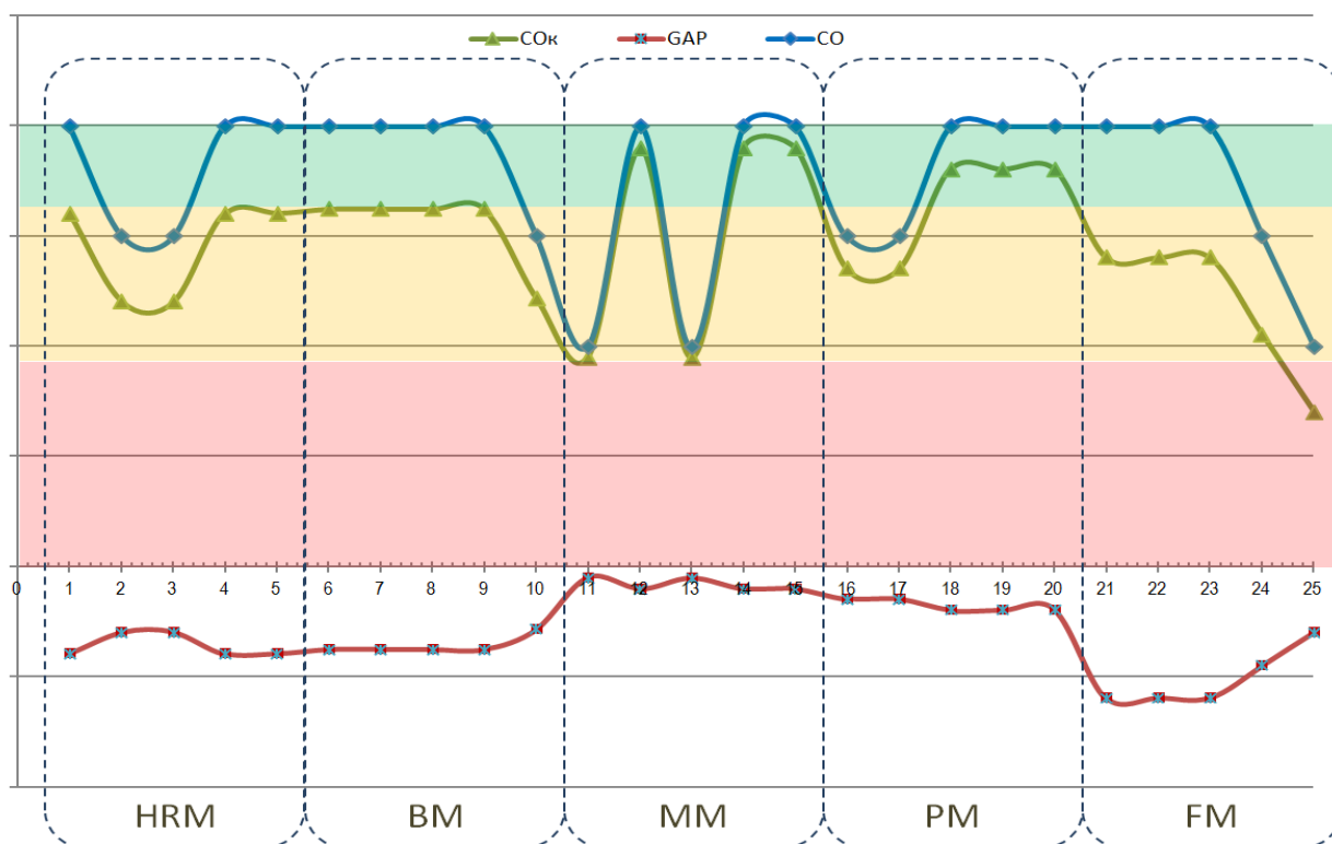
Рис.4. Графики по 25 критериям (по 5 критериев в каждом из 5 факторов): Самооценка (CO), Самооценка скорректированная (COк), GAP
