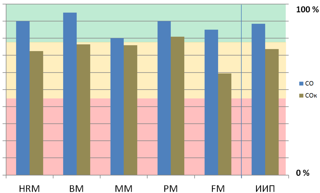
Рис.2. Гистограмма: Самооценка (CO), Самооценка скорректированная (COк), ИИП
